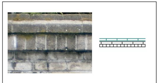
図 19 積み方 K : 中央長手+長手+小口縦 (1 例)
