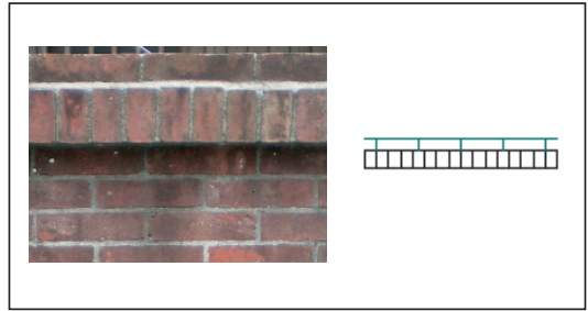
図 17 積み方 I : 中央長手+小口縦並び (4 例)
