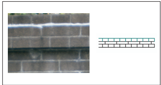
図 18 積み方 J : 中央小口+長手+小口 (1 例)
