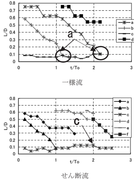
図-3 変動特性
