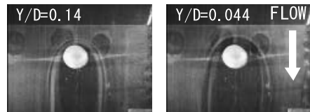
図-4 水平断面形象(case2)
